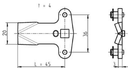
Sluitlip met stangenbediening (vleugellip)
